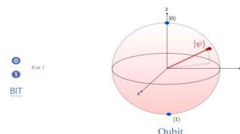
Qubit
